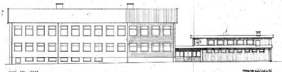
Skolan. Fasad mot söder (Tavelsjövägen) efter tillbyggnad.
