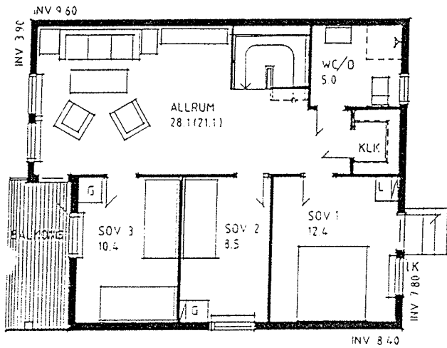
ÖVERPLAN
